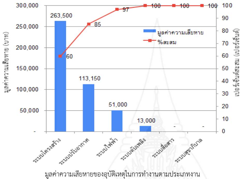
ภาพที่ 1 มูลค่าความเสียหายของอุปกรณ์ในการทำงานตามระบบของงานก่อสร้างปรับปรุงร้านค้าในท่าอากาศยานสุวรรณภูมิ
