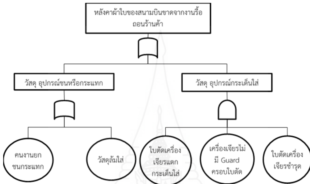
ภาพที่ 4 ความผิดพลาดแบบแผนภูมิต้นไม้ของการเกิดอุบัติเหตุในการรื้อถอนโครงสร้างหลักของอาคารผู้โดยสาร
