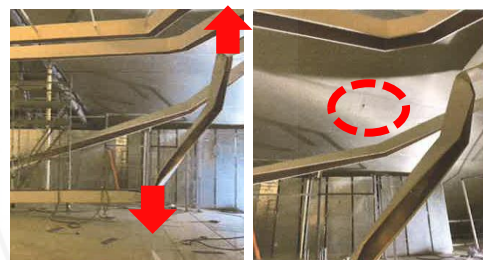
3c) การฉีกขาดของโครงสร้างหลังคาผ้าใบ
